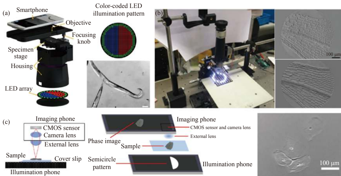
图 18 各种基于智能手机平台的差分相衬显微镜示意图。(a) Jung 等提出的基于智能手机平台的显微镜示意图 [135] ; (b) Ogasawara 等提出的基于智能手机平台的显微镜示意图 [136] 。(c) Kheireddine 等提出的基于智能手机平台的显微镜示意图 [131]
