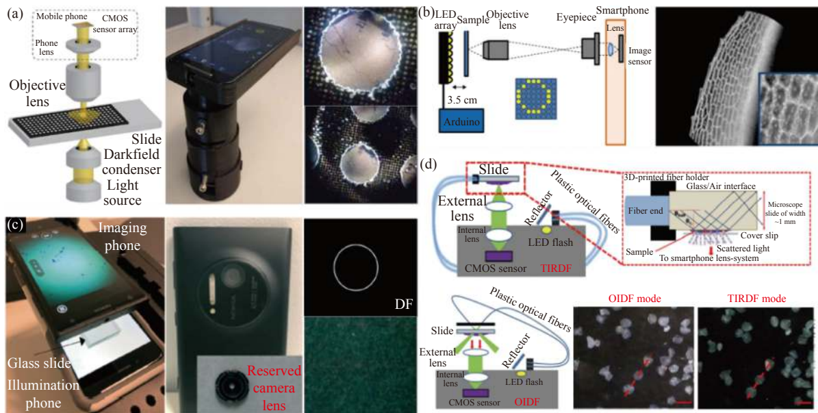
图 17 各种基于智能手机平台的暗场显微镜示意图。(a) Sun 等提出的基于智能手机平台的显微镜示意图 [134] ；(b) Ogasawara 等提出的基于智能手机平台的显微镜示意图 [136] ；(c) Kheireddine 等提出的基于智能手机平台的显微镜示意图 [131] 。(d) Rabha 等提出的基于智能手机平台的显微镜示意图 [116]
