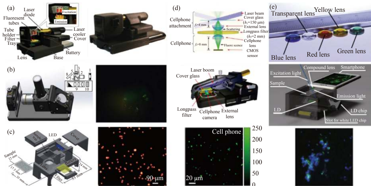
图 20 各种基于智能手机平台的荧光显微镜示意图。(a) Coskun 等提出的基于智能手机平台的显微镜示意图；(b) Cai 等提出的基于智能手机平台的显微镜示意图 [130] ；(c) Zhu 等提出的基于智能手机平台的显微镜示意图 [162] ；(d) Wei 等提出的基于智能手机平台的显微镜示意图 [95] ；(e) Dai 等提出的基于智能手机平台的显微镜示意图 [163]
