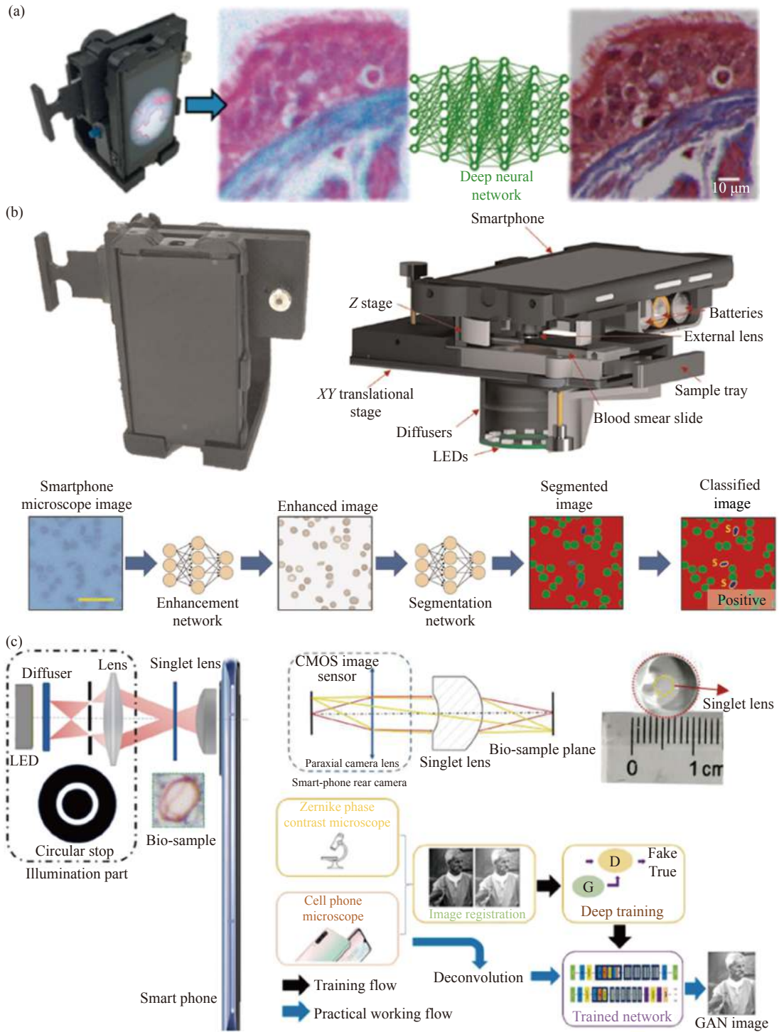
图 15 各种结合深度学习的基于智能手机平台的显微镜。(a) Rivenson 等提出的智能手机显微镜系统结构和深度学习结果示意图 [120] ；(b) Haan [121] 等提出的智能手机显微镜系统结构示意图和两个深度学习网络的工作流程图 [121] ；(c) Bian [119] 等提出的智能手机显微镜系统结构示意图和基于深度学习风格迁移方法的工作流程图
