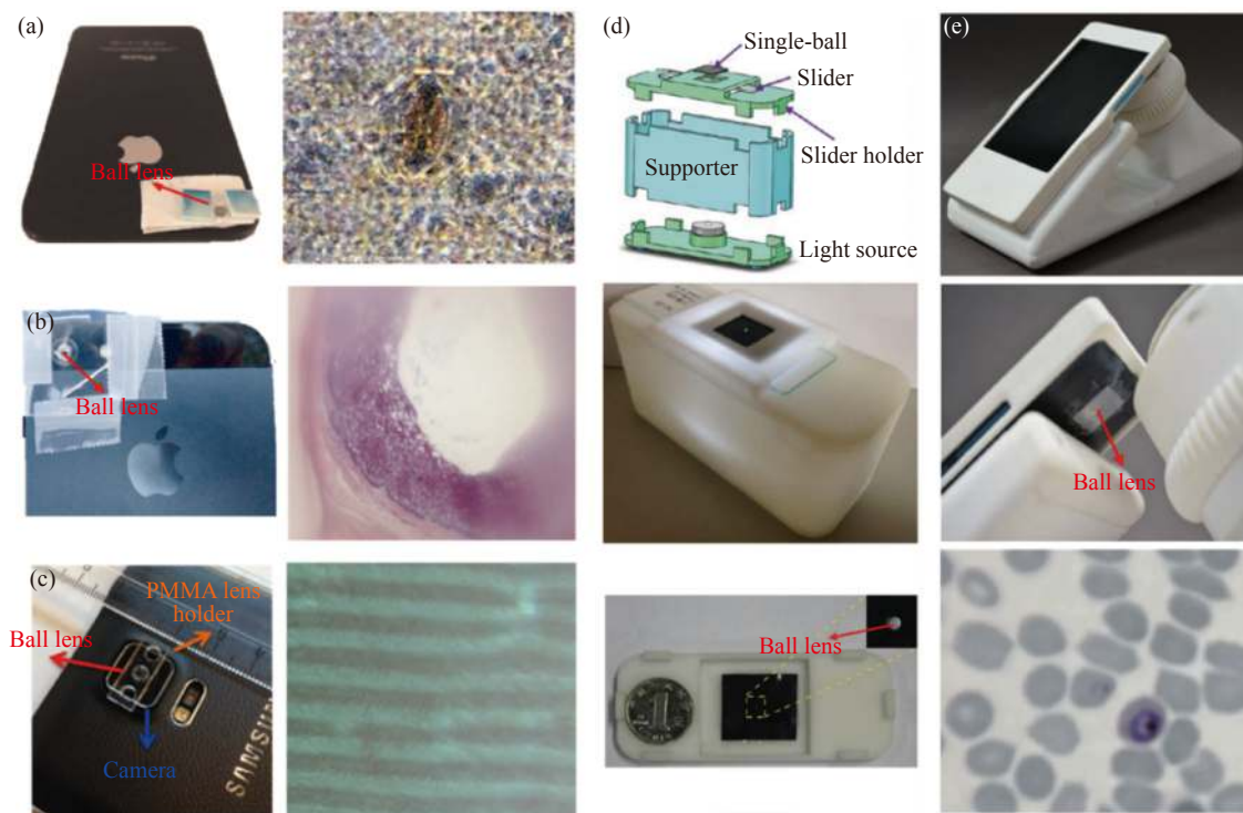
图 4 各种基于球透镜的智能手机平台显微成像系统示意图。(a) Bogoch 提出的基于智能手机平台的显微镜示意图 [62] ; (b) Jahan-Tigh 等提出的基于智能手机平台的显微镜示意图 [42] ; (c) Kutay 等提出的基于智能手机平台的显微镜示意图 [65] ; (d) Zeng 等提出的基于智能手机平台的显微镜示意图 [63] ; (e) Agbana 等提出的基于智能手机平台的显微镜示意图 [64]
